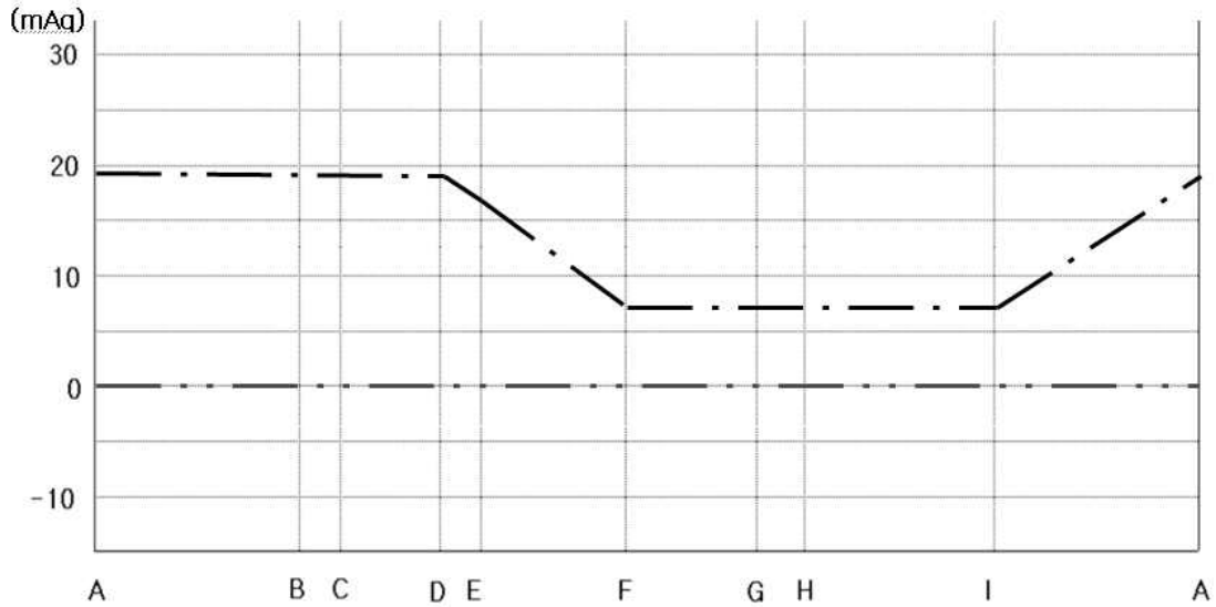
- 난방배관 압력분포도 -
