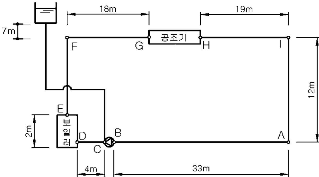
- 난방배관 계통 -
