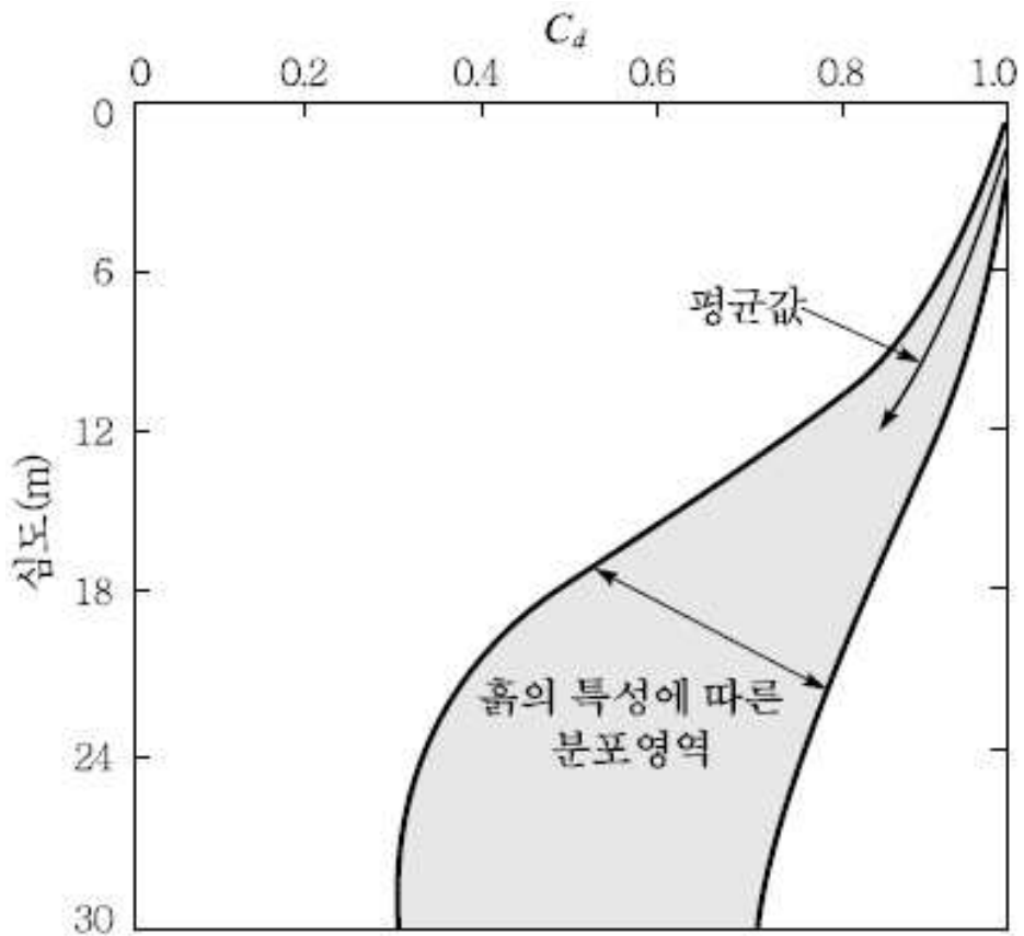
<심도와 동적 전단응력 감소계수 관계곡선(Seed & Idriss, 1987)>
